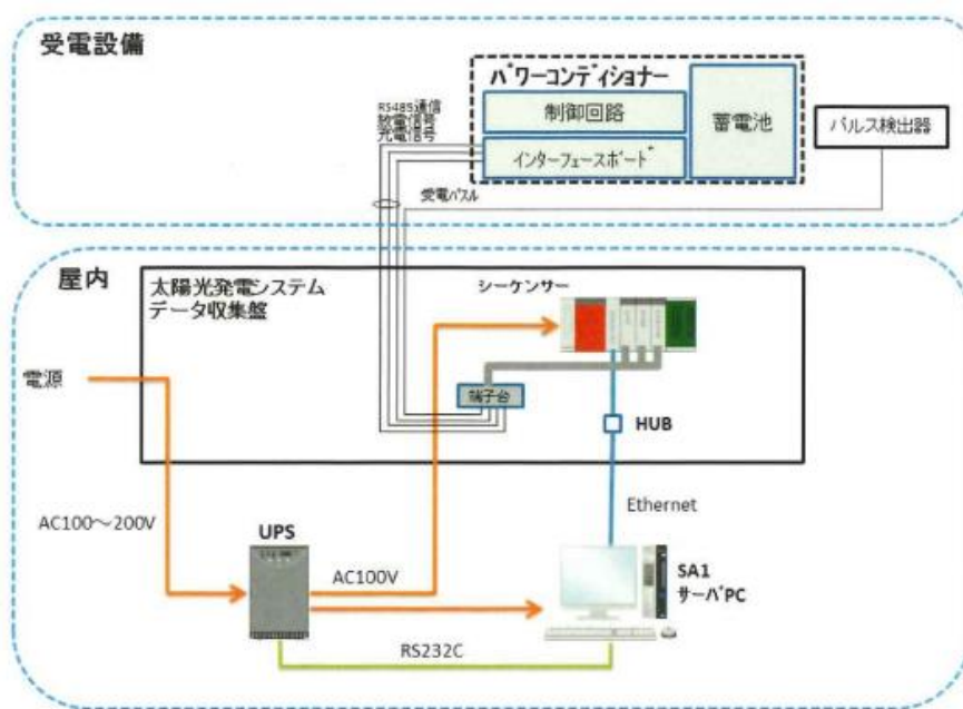
図 2.1 SA1 システム構成図
